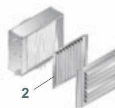
Kit double déflexion sur AZN et AZN-F en montage vertical 0011-30 à 38
